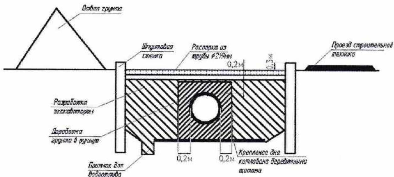
Котлован с устройствами усиления стенок
