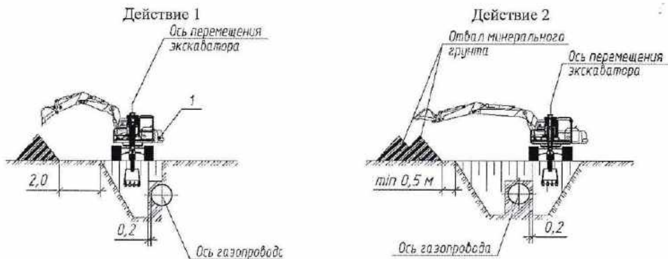
Схема разработки траншеи экскаватором
